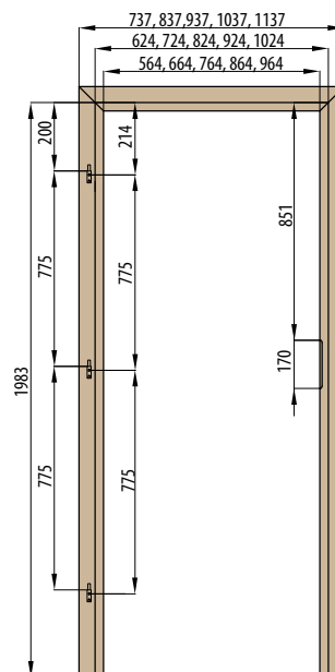
OBKLAD KOVOVÉ ZÁRUBNĚ
